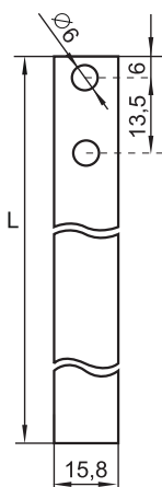
# 14.04.181 L - 500 mm - 2,70 евро # 14.04.185 L - 600 mm - 2,70 евро # 14.04.190 L - 700 mm # 14.04.200 L - 800 mm # 14.04.221 L - 1200 mm - 5,10 евро # 14.04.230 L - 1300 mm
